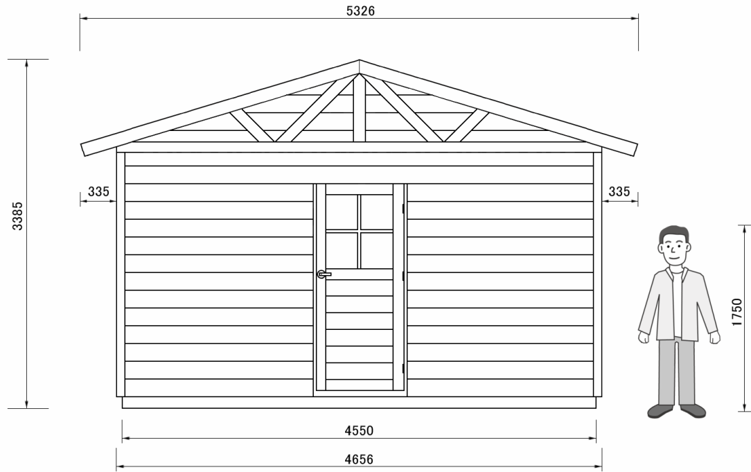
正面图
