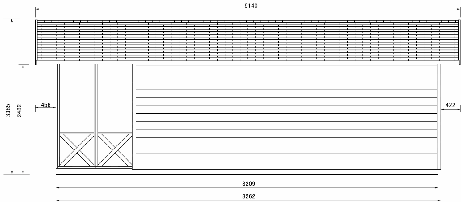
侧面图
