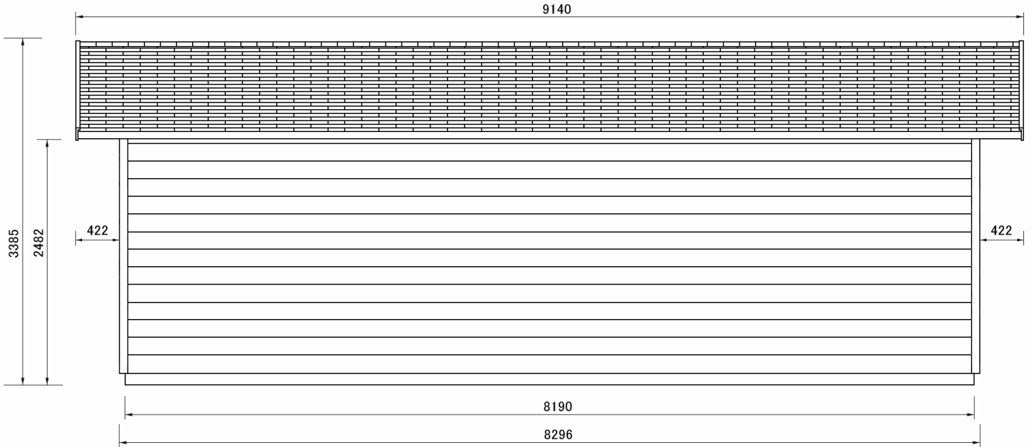
側面図
