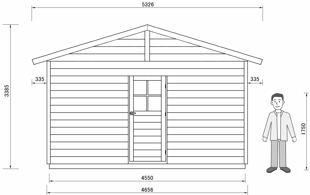
正面図
