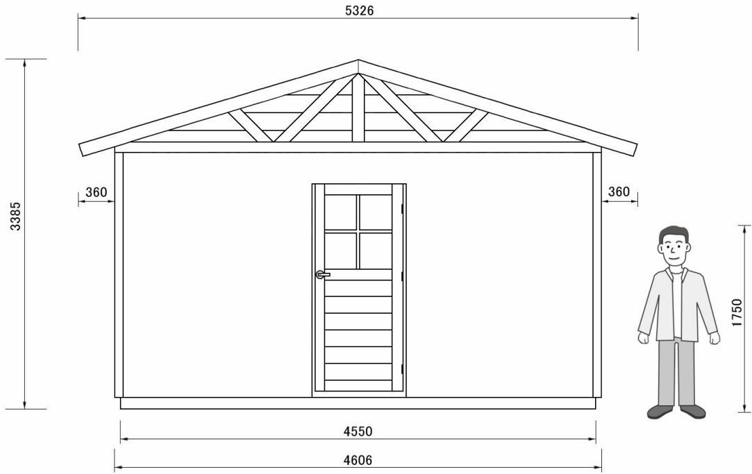
正面图
