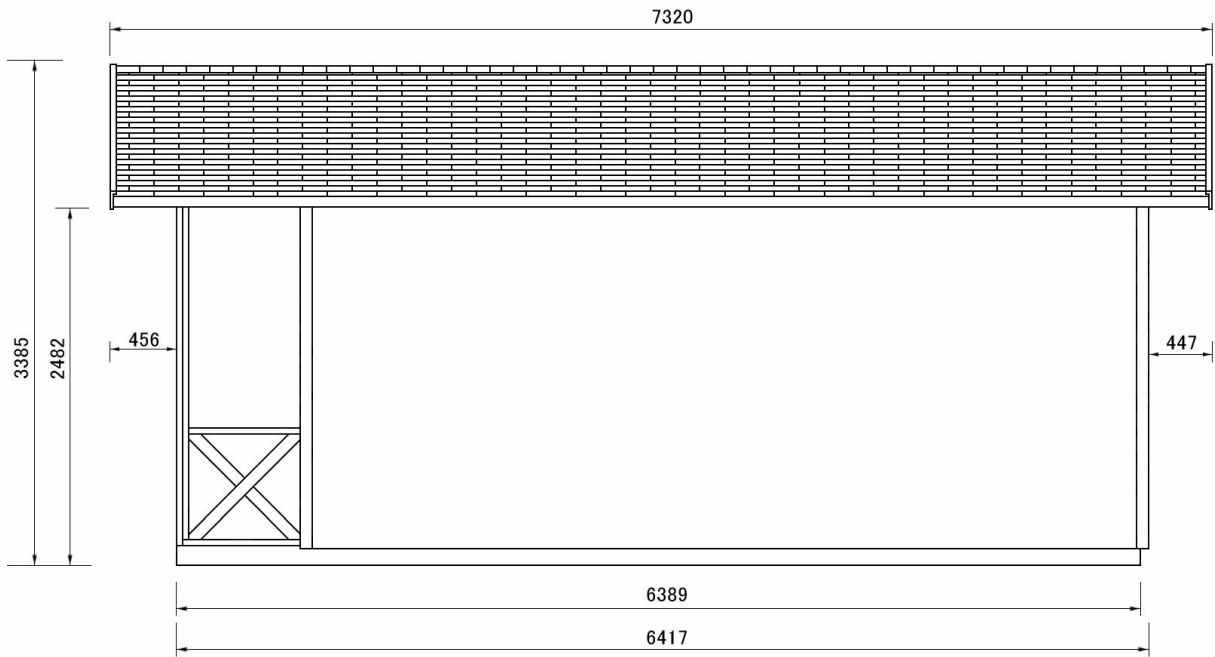
侧面图
