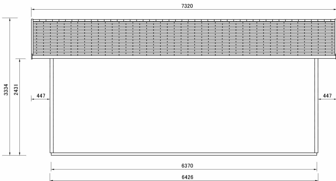
側面図
