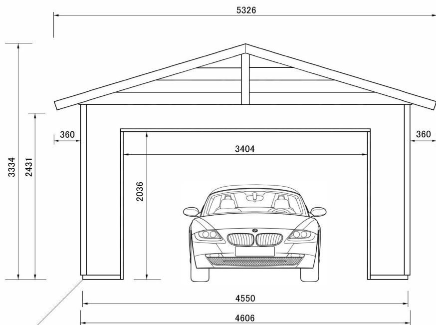
正面図
