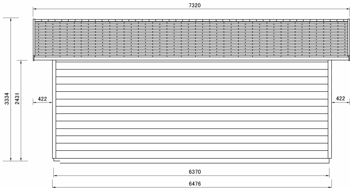
側面図
