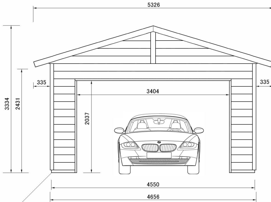
正面図
