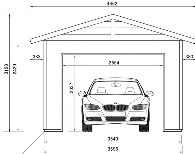
正面図
