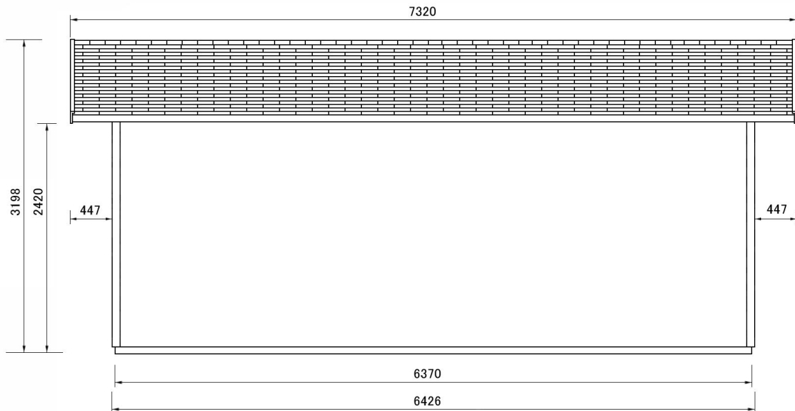
側面図
