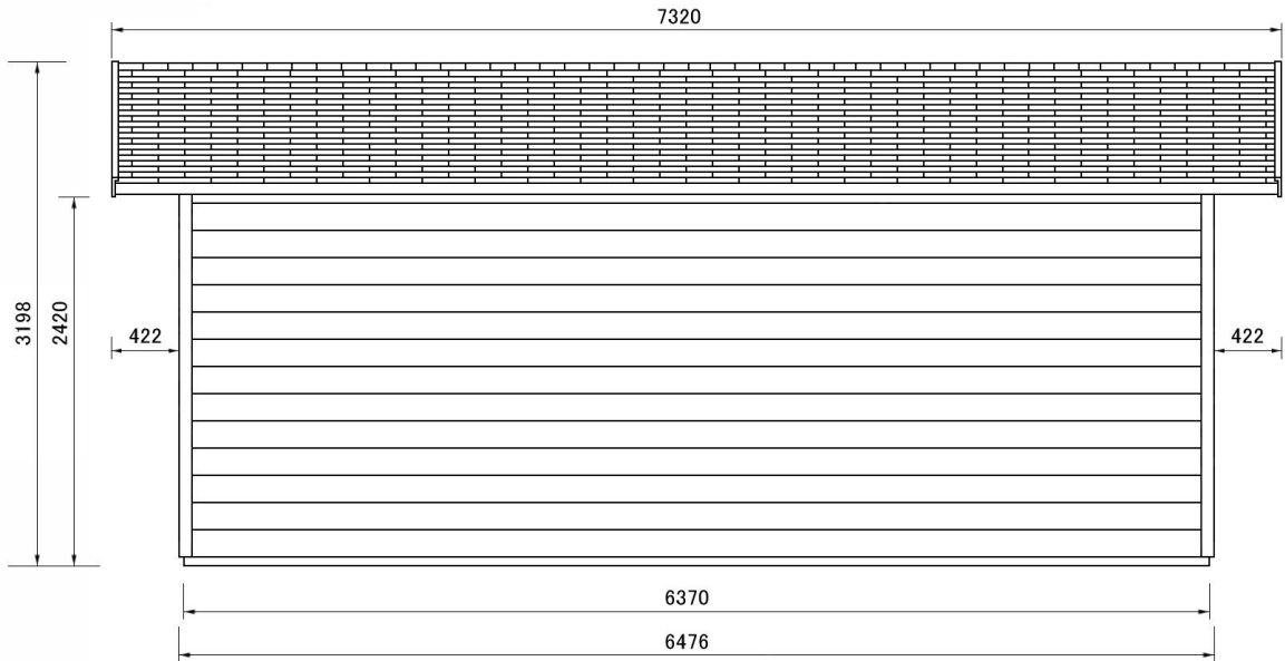
側面図
