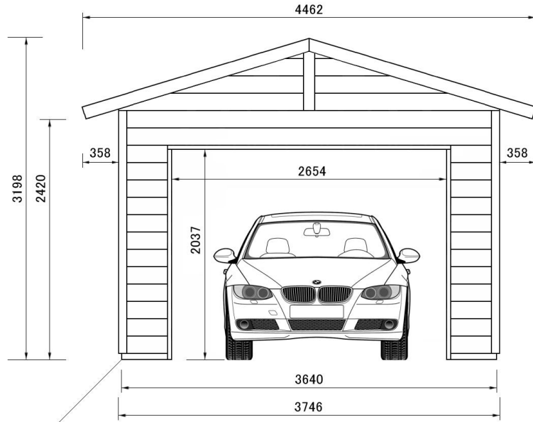
正面図
