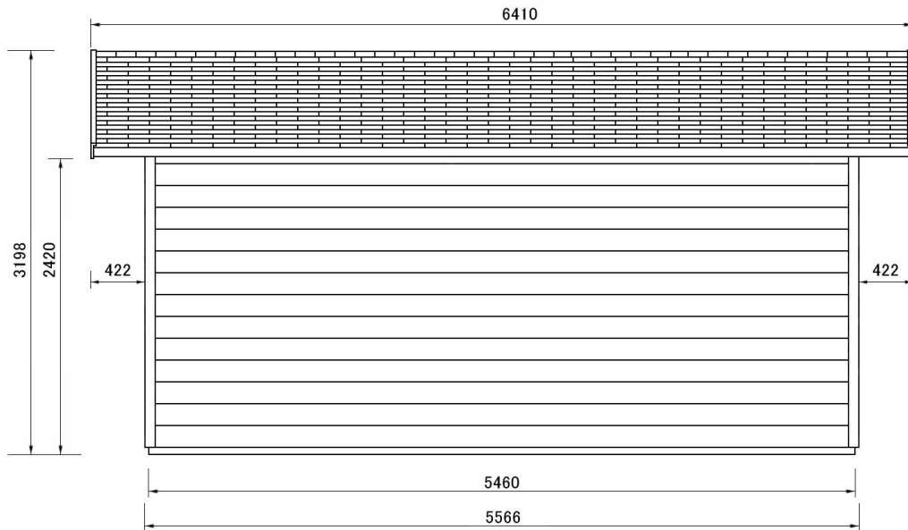
側面図
