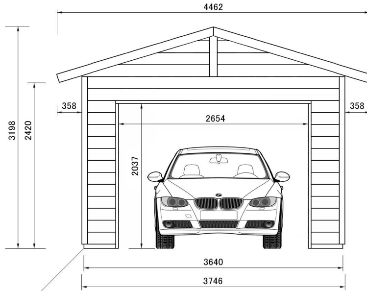
正面図
