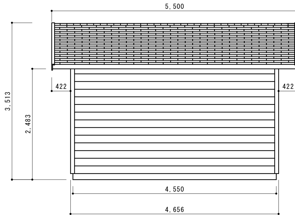
側面図
