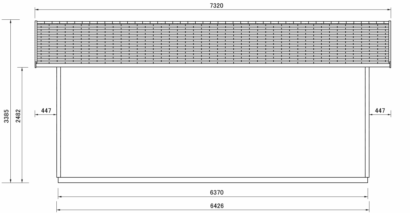
侧面图
