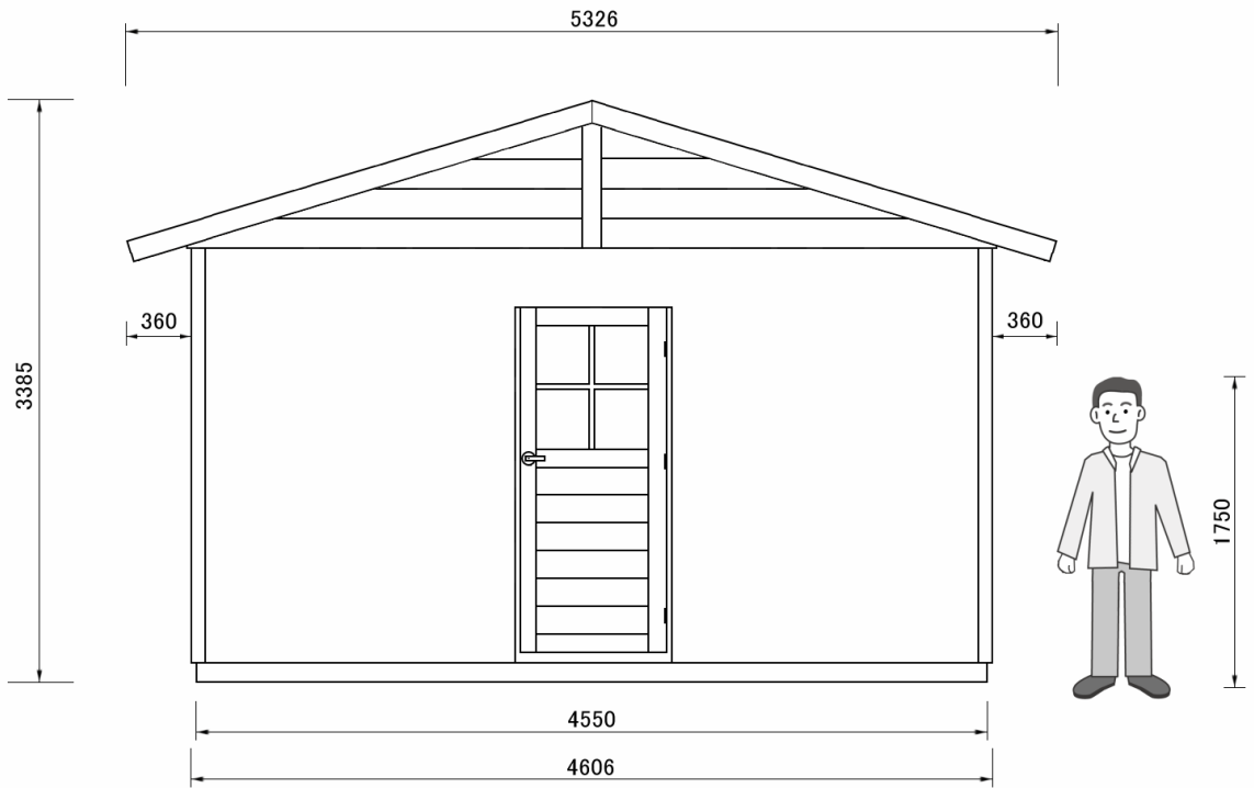
正面图
