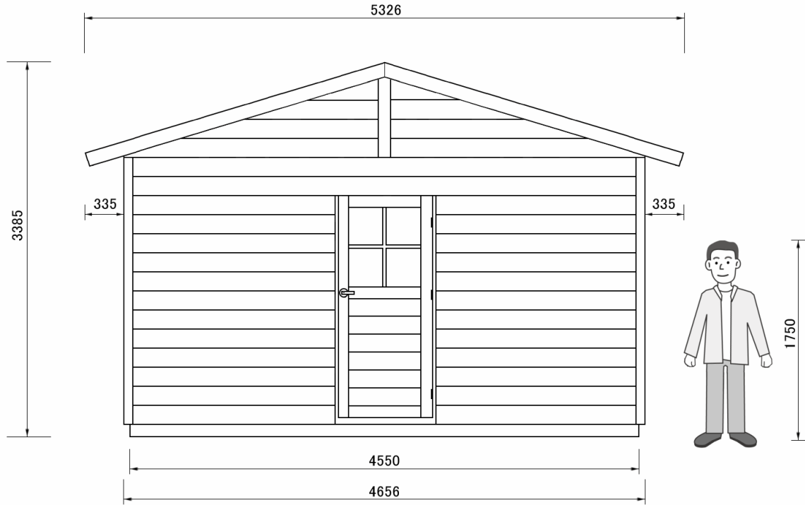
正面图
