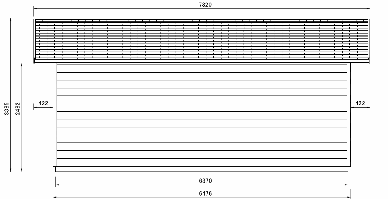
侧面图
