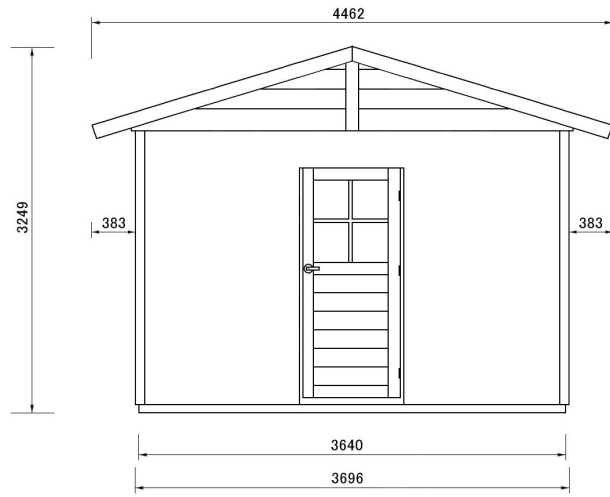
正面图
