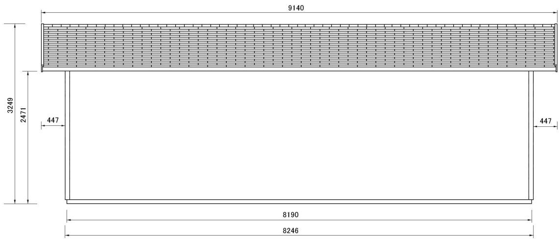
侧面图
