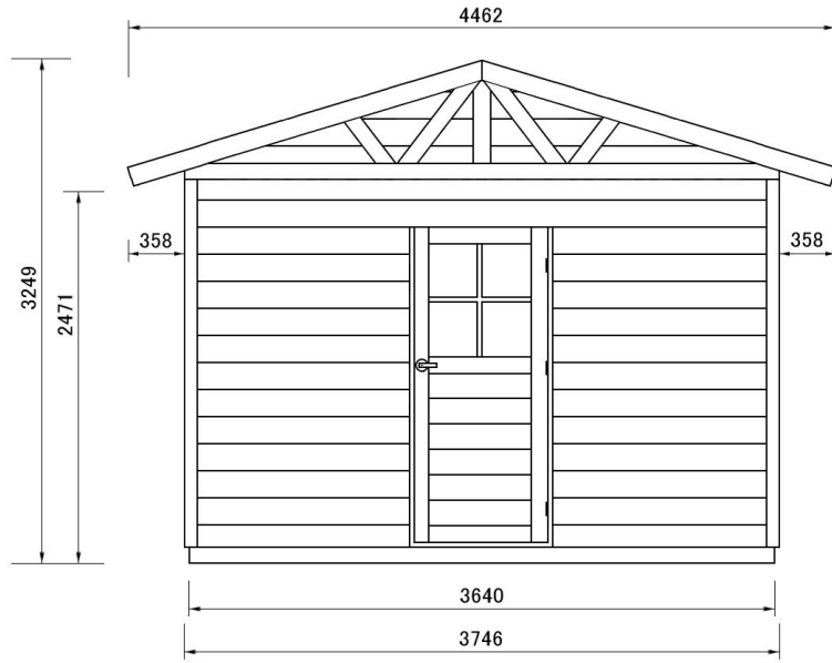
正面图
