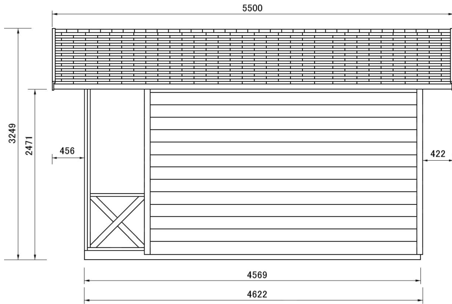
侧面图
