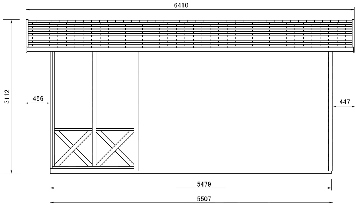
侧面图
