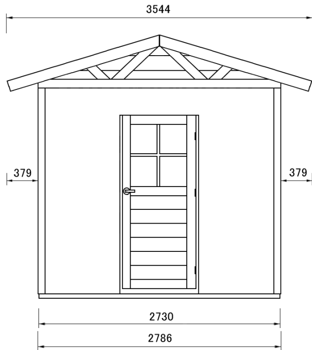
正面图
